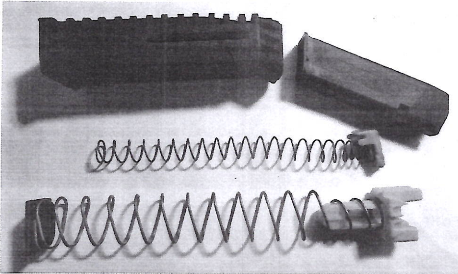
Abbildung 2: Schmeisser Magazinadapter, mit Glock-Magazingehäuse und zweigeteilter Magazinfeder
